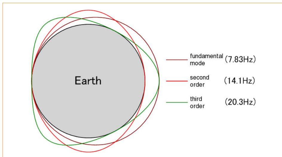
▲ 地球大气层的舒曼共振（Schumann Resonance），基模频率为 7.83 赫兹。
