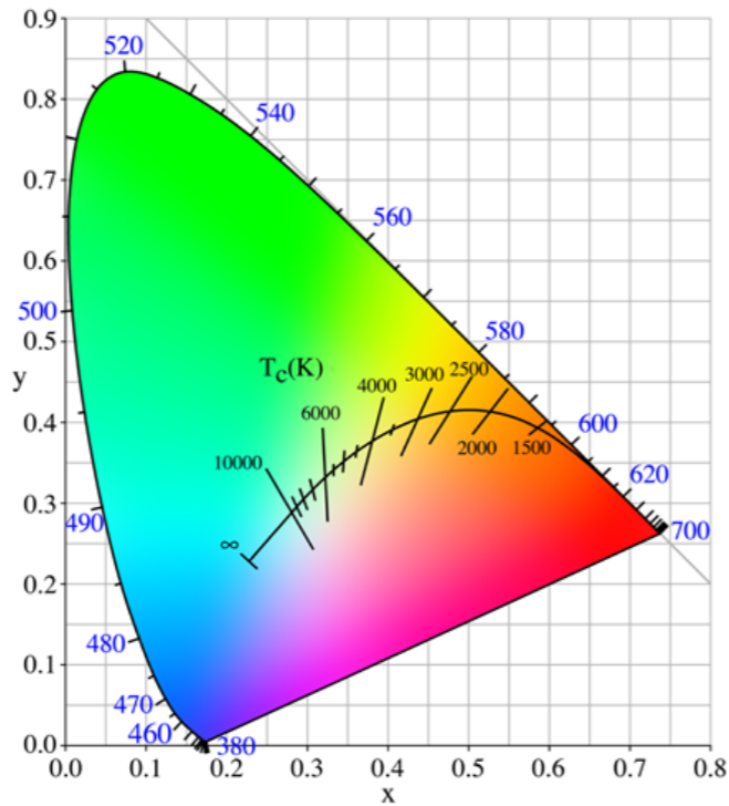
图例：图中整个彩色图形的部份叫作色彩空间，属于人眼可以感知的色彩范围，由国际照明委员会（CIE）于一九三一年制定。彩图中间从红色区域划向蓝色区域的轨迹曲线叫作「普朗克轨迹」，曲线上的数字刻度表示辐射源的温度。
