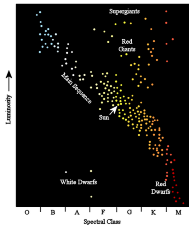
图例：这幅示意图（赫罗图）展示了恒星的光度与色彩，我们看到恒星的色彩整体分为红、橙、黄、白、蓝白、蓝几色。
